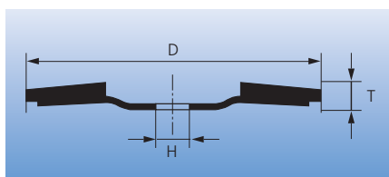
Ejecución cónica
